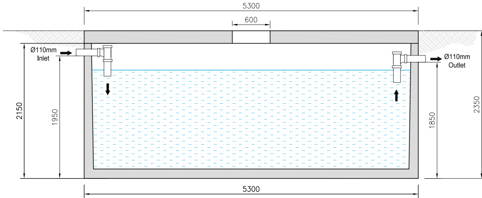
Section A-A
