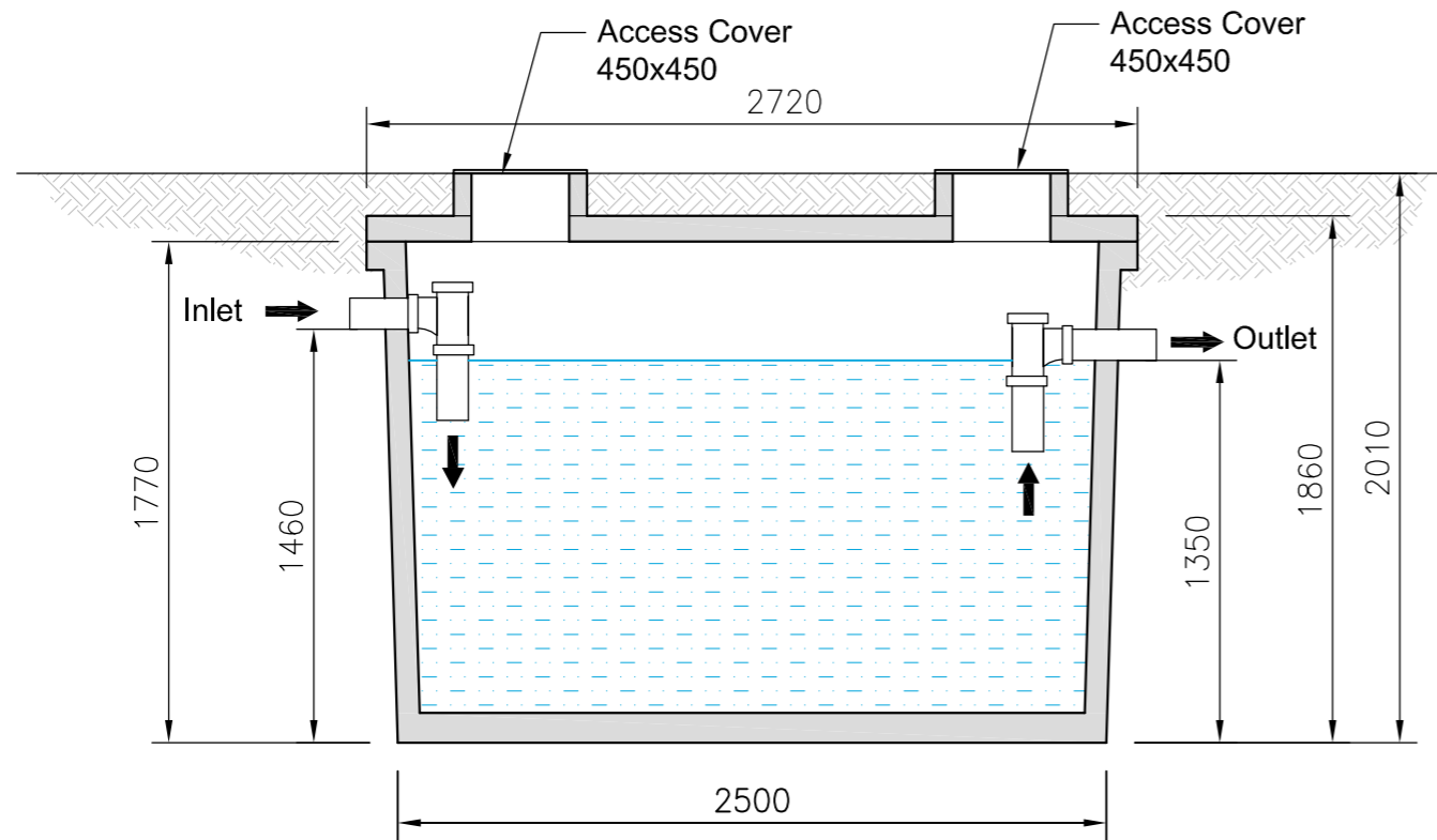
Section A-A
