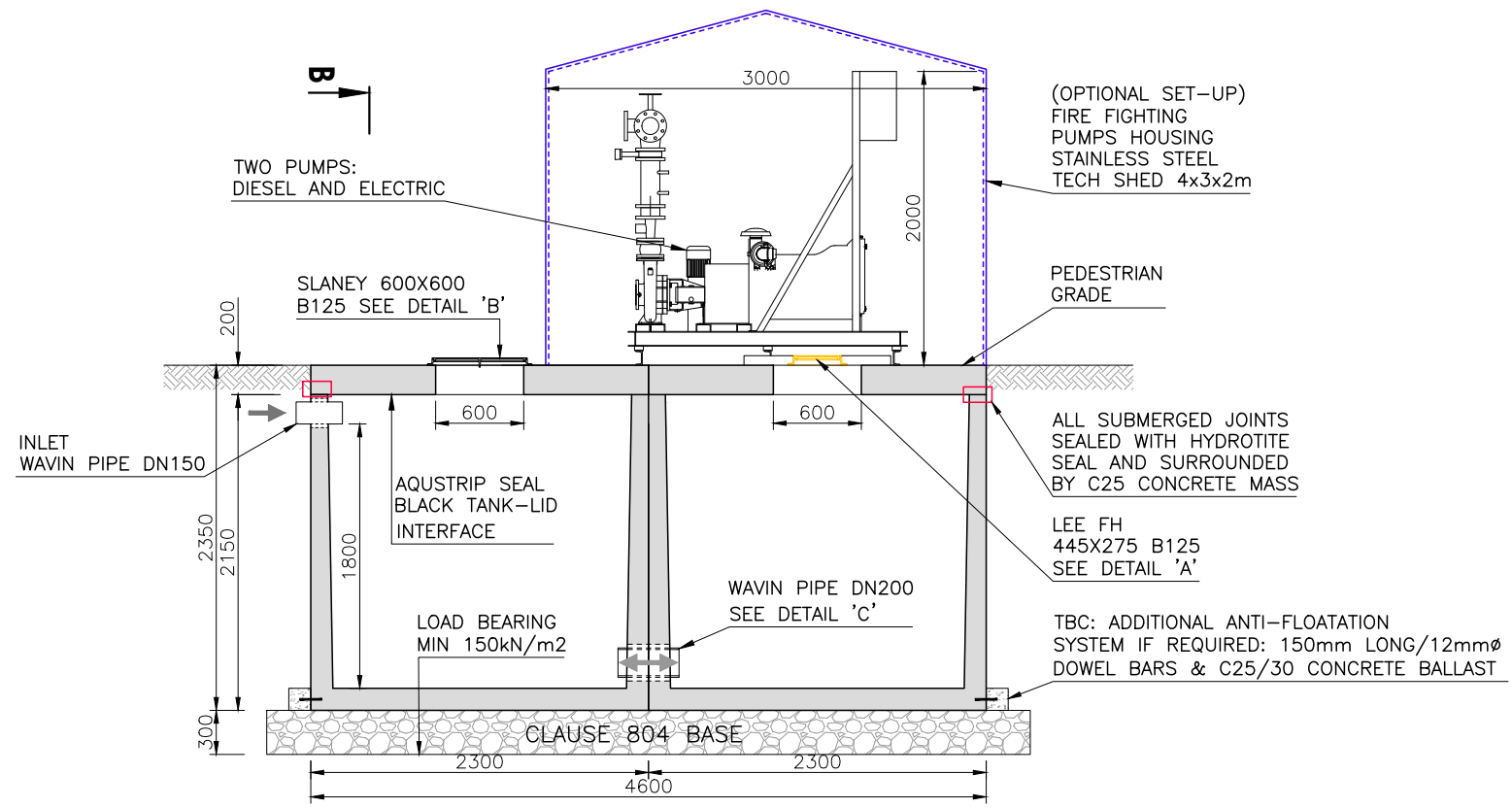
SECTION A-A 1:50 @ A3
