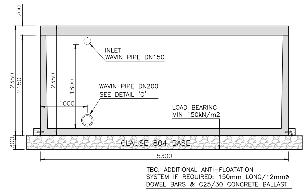
SECTION B-B 1:50 @ A3
