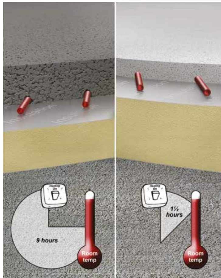
Sand:Cement Screed
